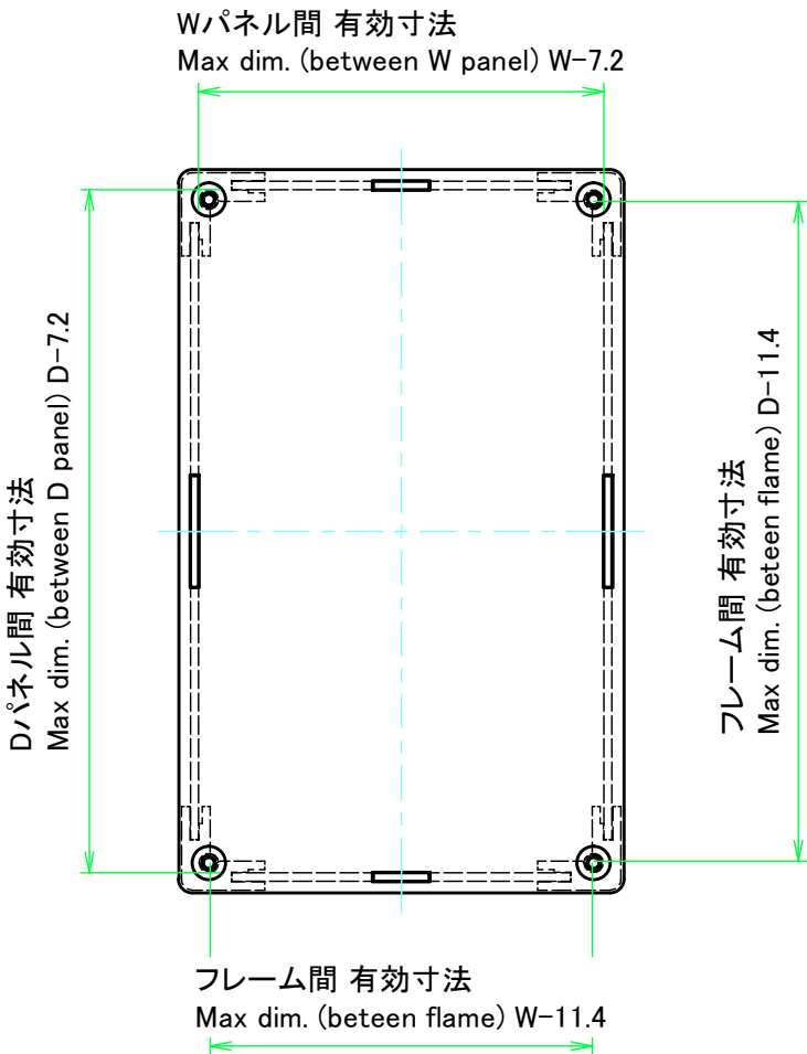
下カバー / Bottom cover
